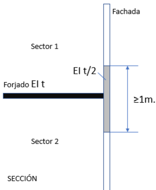
Figura 2.9: Compartimentación vertical.
